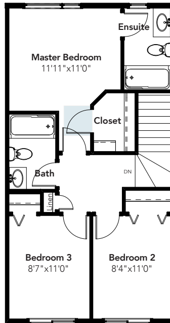
CLOSET DOOR
