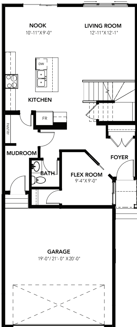
MAIN: 832 SQ FT
